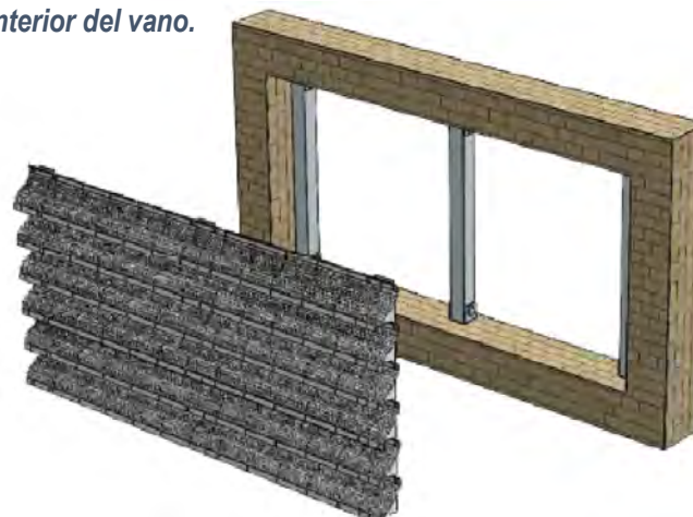
Instalación en interior del vano.
