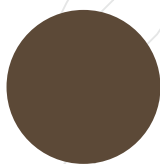
ASTEROIDE
