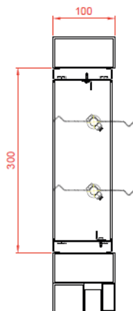
SECCION ALETAS
