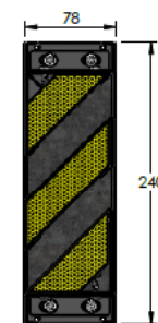
SECCIÓN A-A
